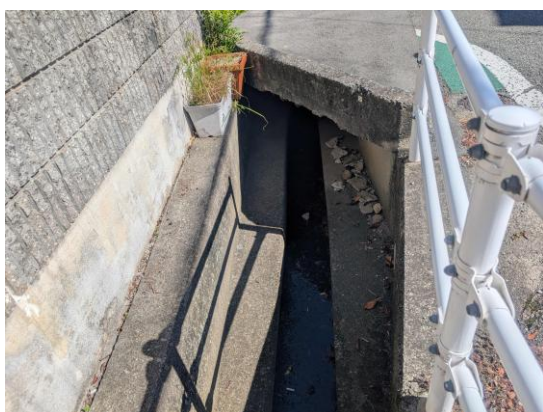
左写真:破損状況(工事前)
